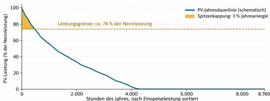
Abbildung 1: Schematische PV-Jahresdauerlinie. Die Begrenzung seltener Einspeisespitzen auf 74% der Höchst einspeiseleistung reduziert die erforderliche Netzleistung und generiert beispielhaft nur einen Verlust von 3 % der Jahresenergiemenge. Bei 74% Leistung werden 97% der Energiemenge eingesammelt.
